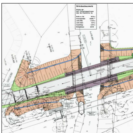
Auszug aus Lageplan Brückenbauwerk
