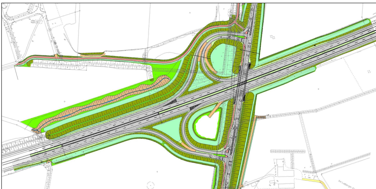
Lageplan BAB-Anschlussstelle
