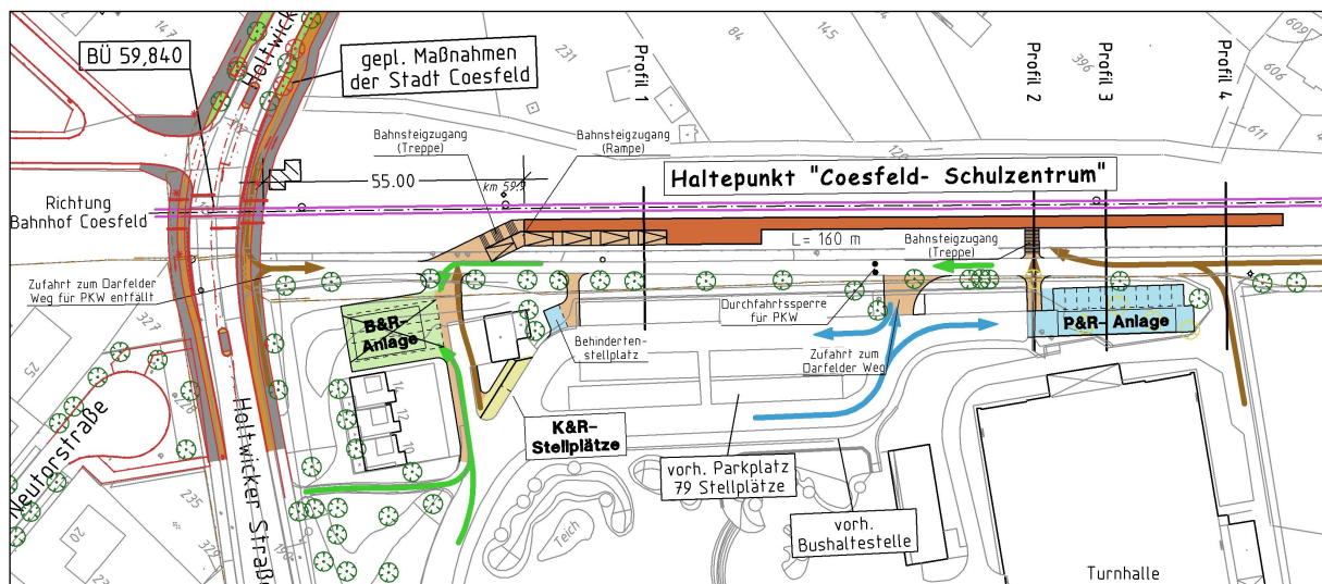
Lageplanausschnitt
