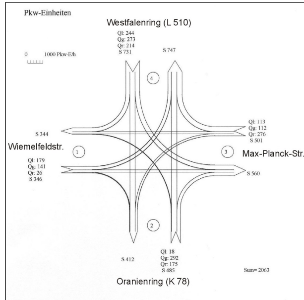
Verkehrsuntersuchung
