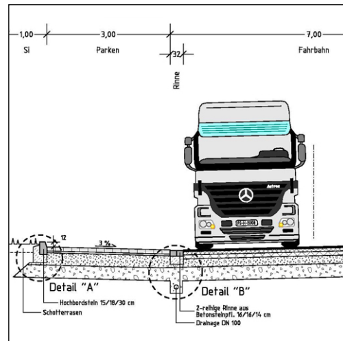
Ausbauquerschnitt
