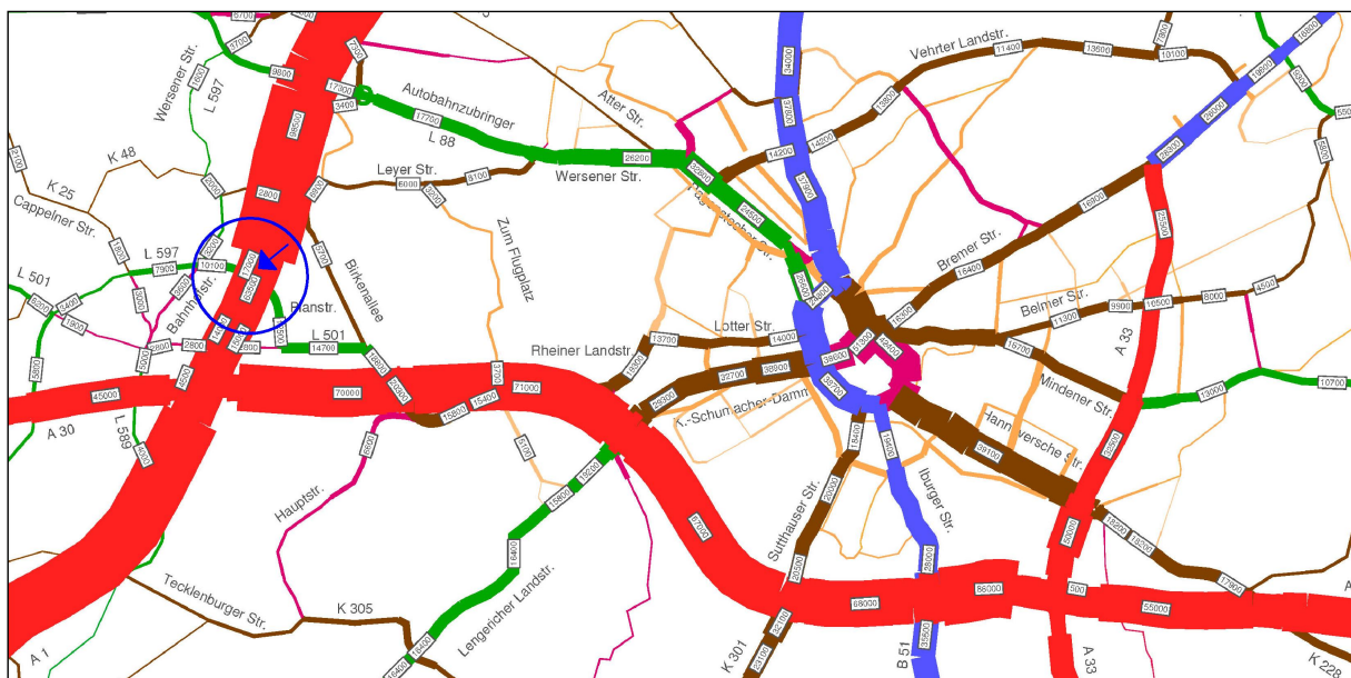
Netzbelastungsplan (Prognose-Planfall mit neuer AS an BAB A 1)
