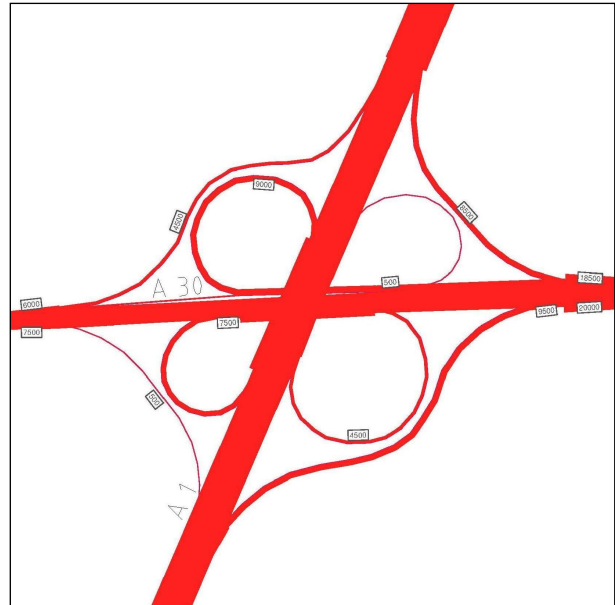
Knotenstrombelastung „Lotter Kreuz“ – Prognose 2020
