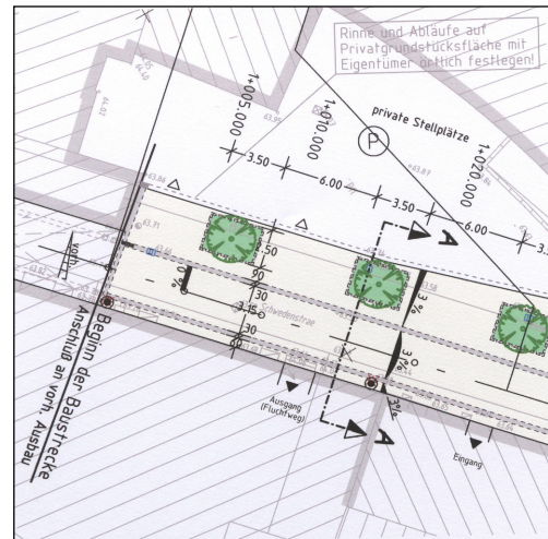
Lageplan
