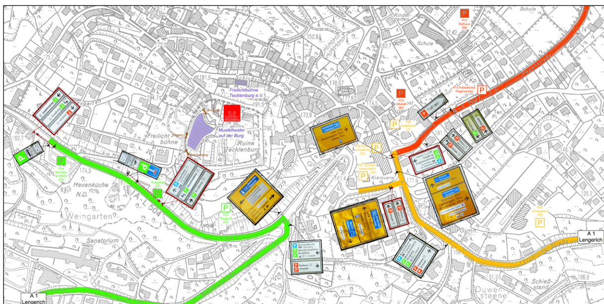
Beschilderungsplan zum Parkleitsystem
