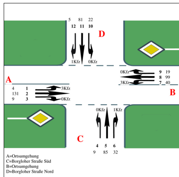
Ausschnitt: Leistungsfähigkeitsberechnung
