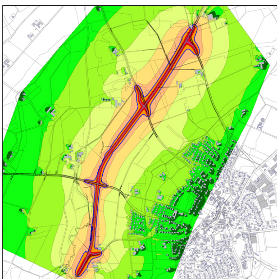
Rasterlärmkarte: Verkehrslärmprognose 2025
