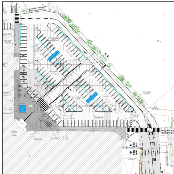
Bauabschnitt Hauptparkplatz
