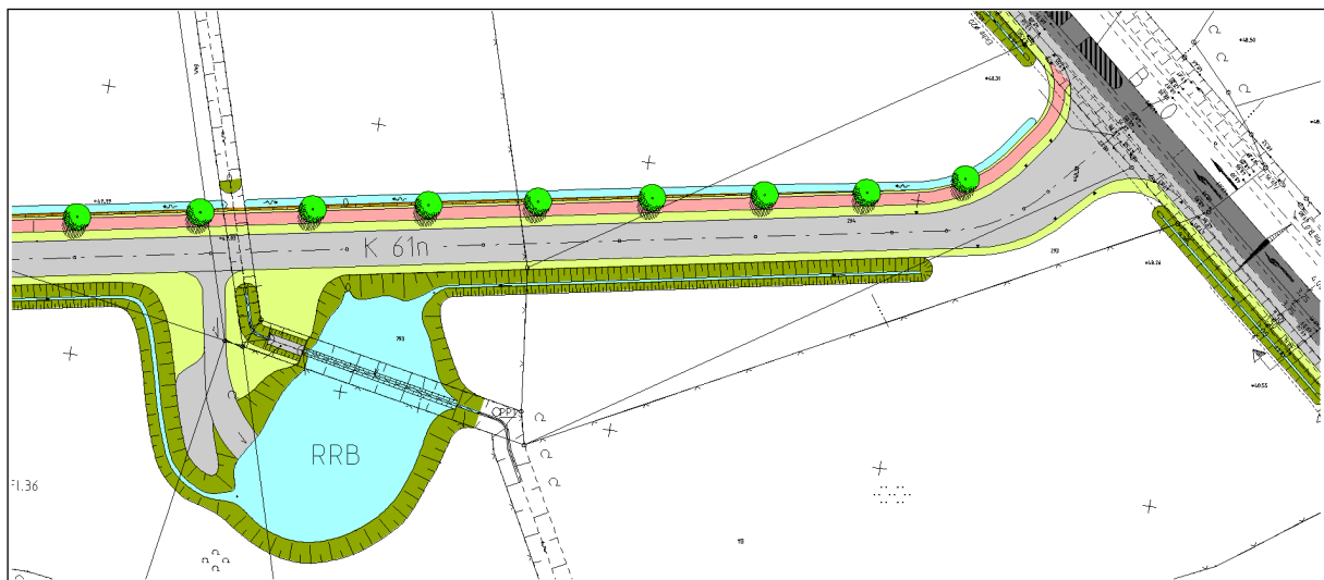
Lageplanausschnitt mit Rückhaltebecken
