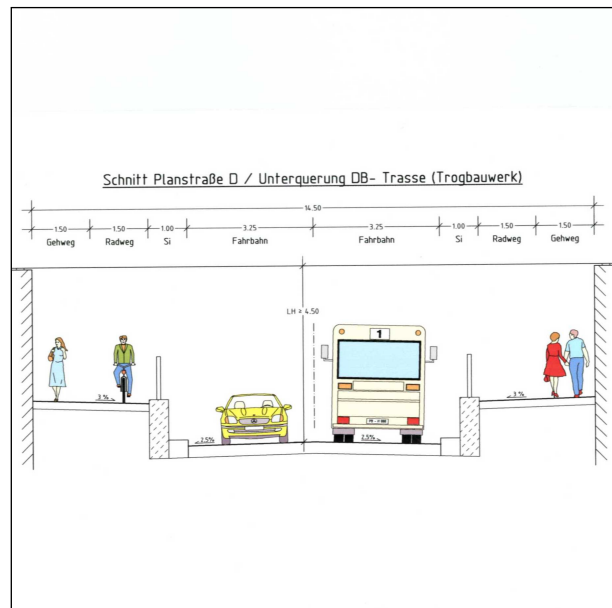
Querschnitt im Bereich der Eisenbahnunterquerung
