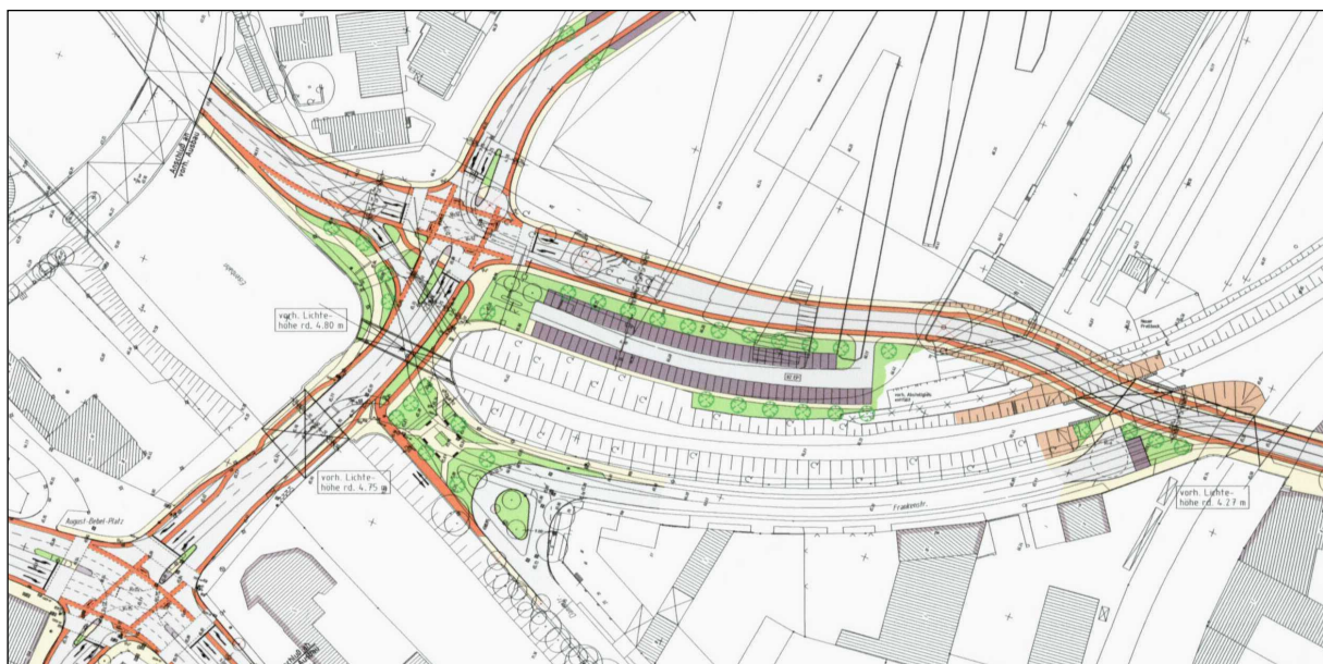
Lageplan Verlegung der Frankenstraße
