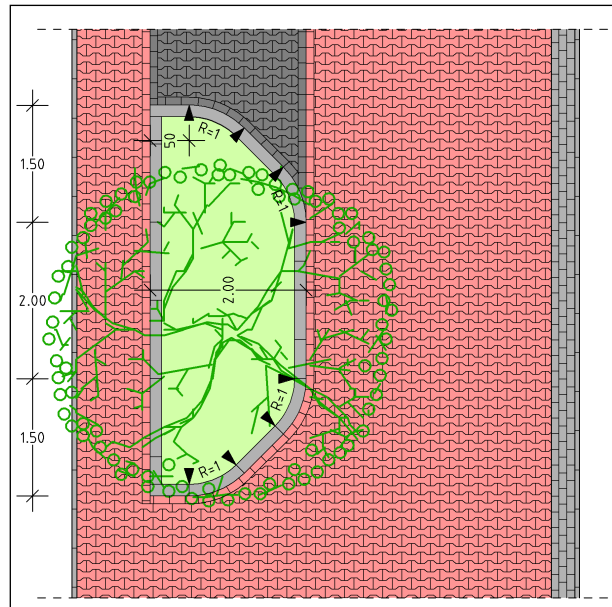
Detail Pflanzbeet
