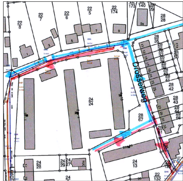
Ausschnitt Konzept Kanalplanung
