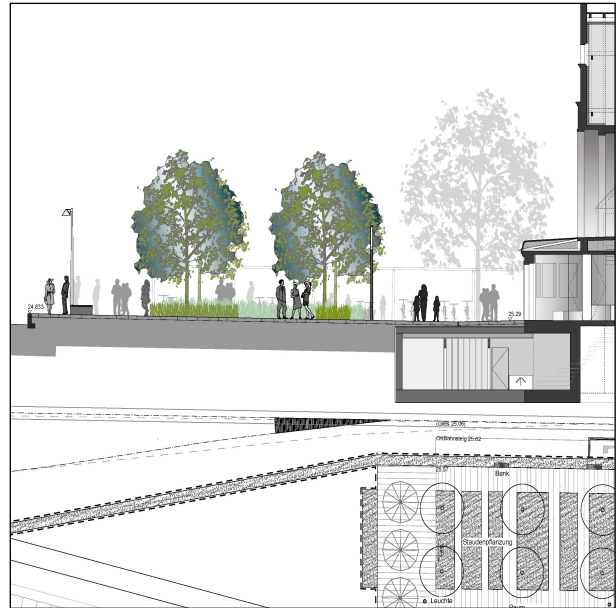
Schnitt
