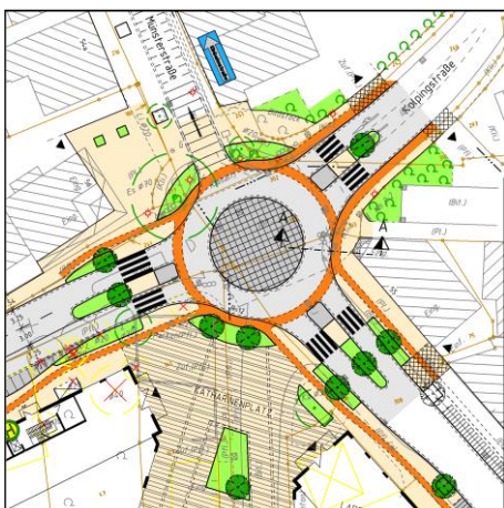
Neubau Kreisverkehrsplatz mit Anschluss an die vorh. Geschäftsstraße
