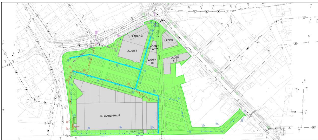
Lageplan mit Kanalisation
