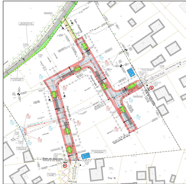
Entwässerung eines Erschließungsgebietes
