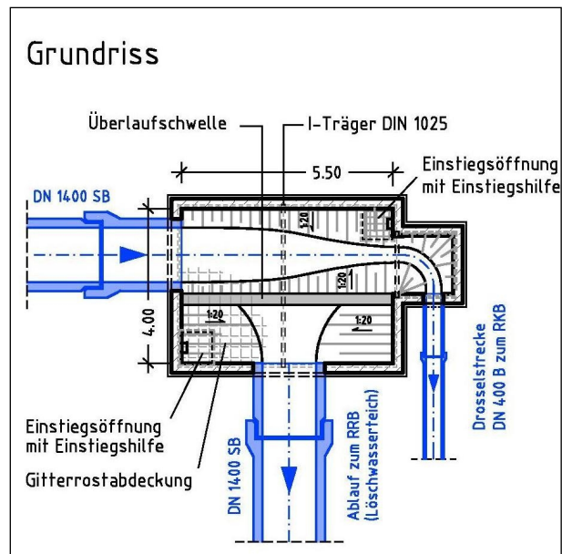
Trennbauwerk
