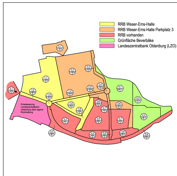
Übersichtsplan Einzugsgebiete
