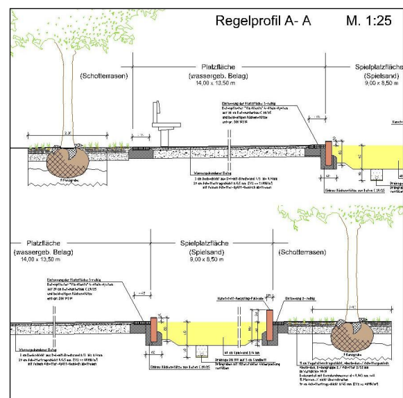
Querschnitt durch Platz
