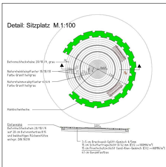
Ausführungsdetail Sitzplatzrondell
