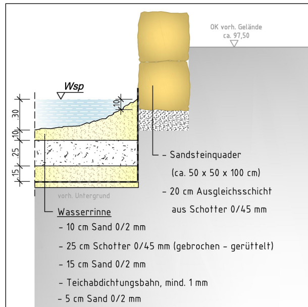
Detail Wasserlauf
