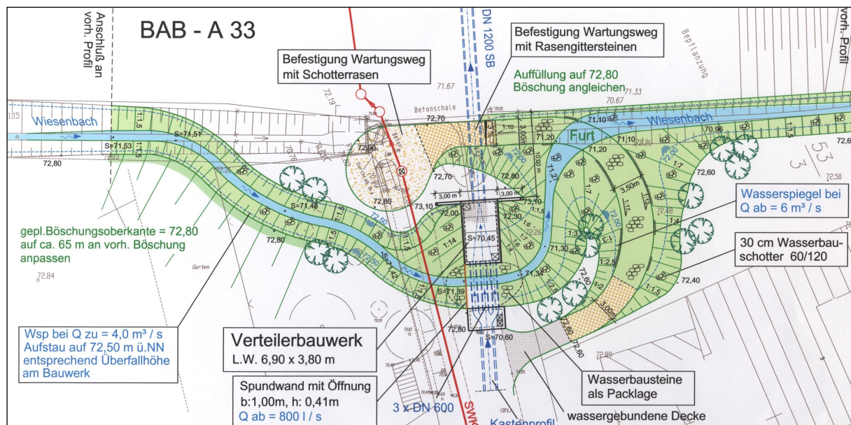
Lageplanausschnitt
