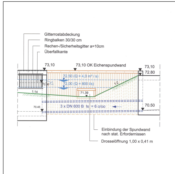
Ansicht Drosselbauwerk
