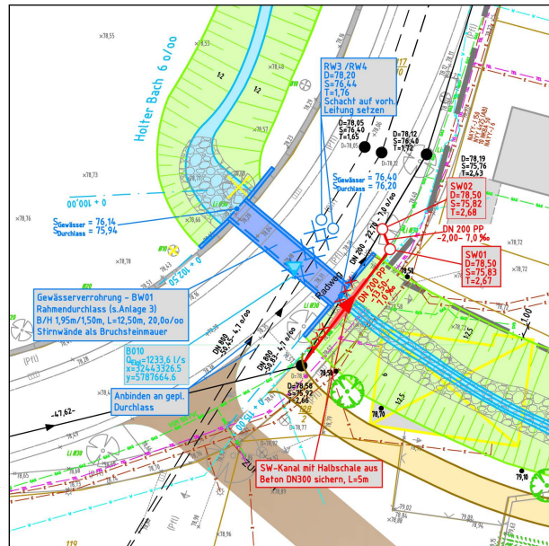
Lageplan
