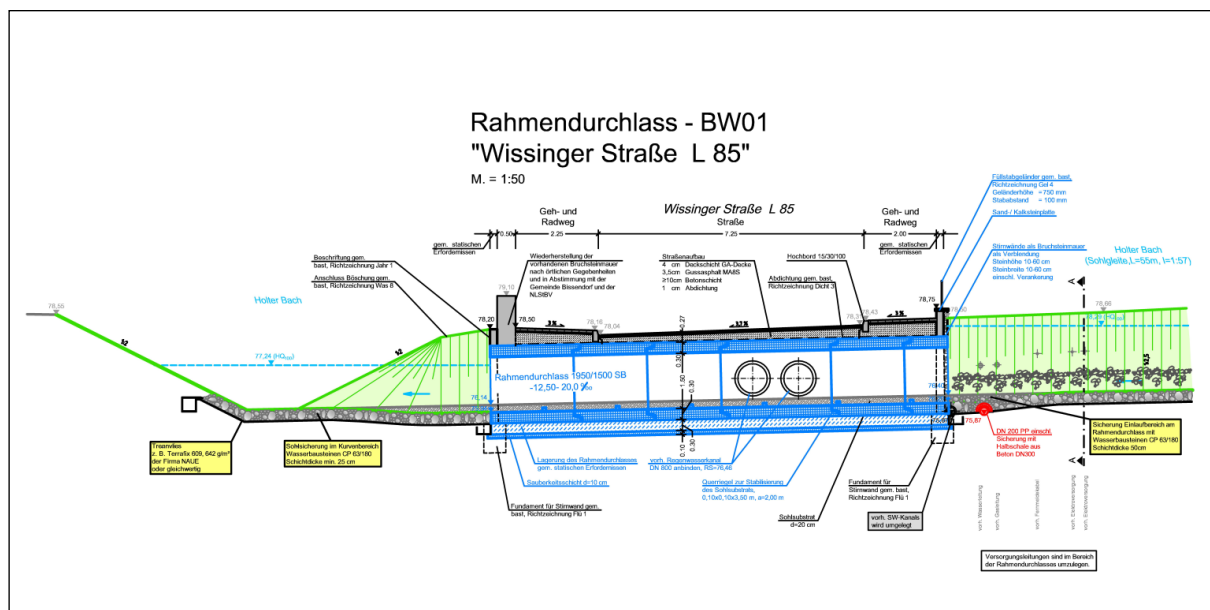
Durchlass
