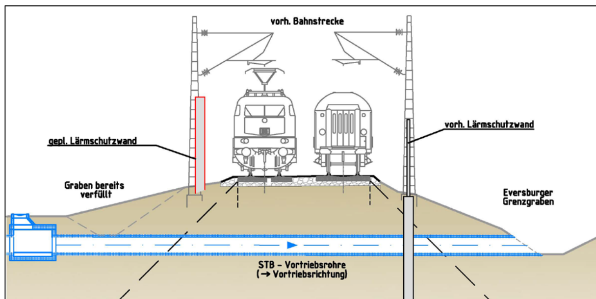
Schnitt Bahnkreuzung
