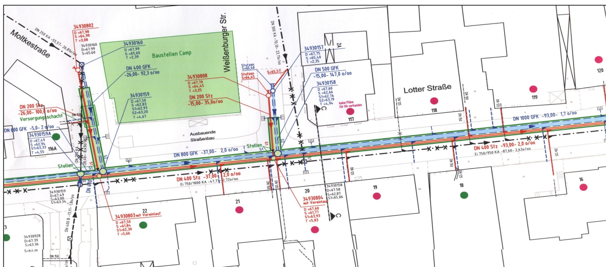
Lageplanausschnitt Lotter Straße
