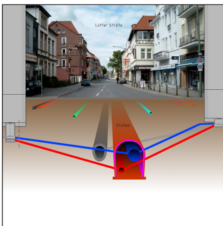
Querschnitt Lotter Straße
