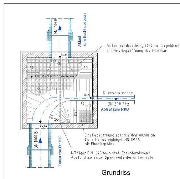
Trennbauwerk
