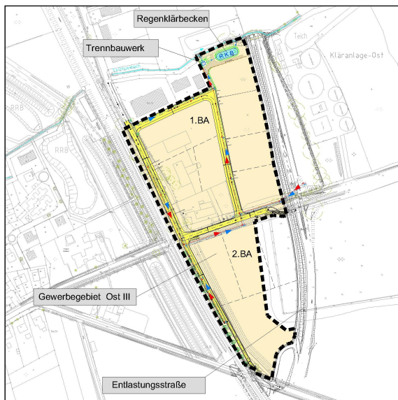
Ausschnitt Übersichtslegeplan
