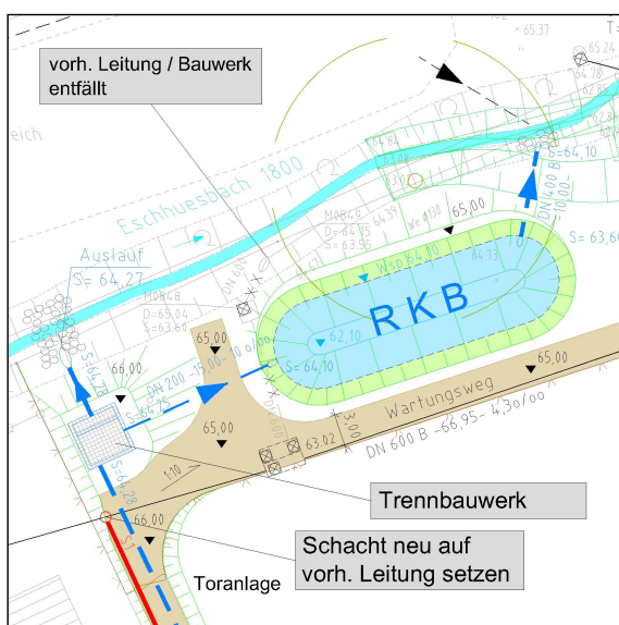
Lageplanausschnitt Regenklärbecken
