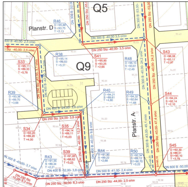
Ausschnitt Lageplan Entwässerung
