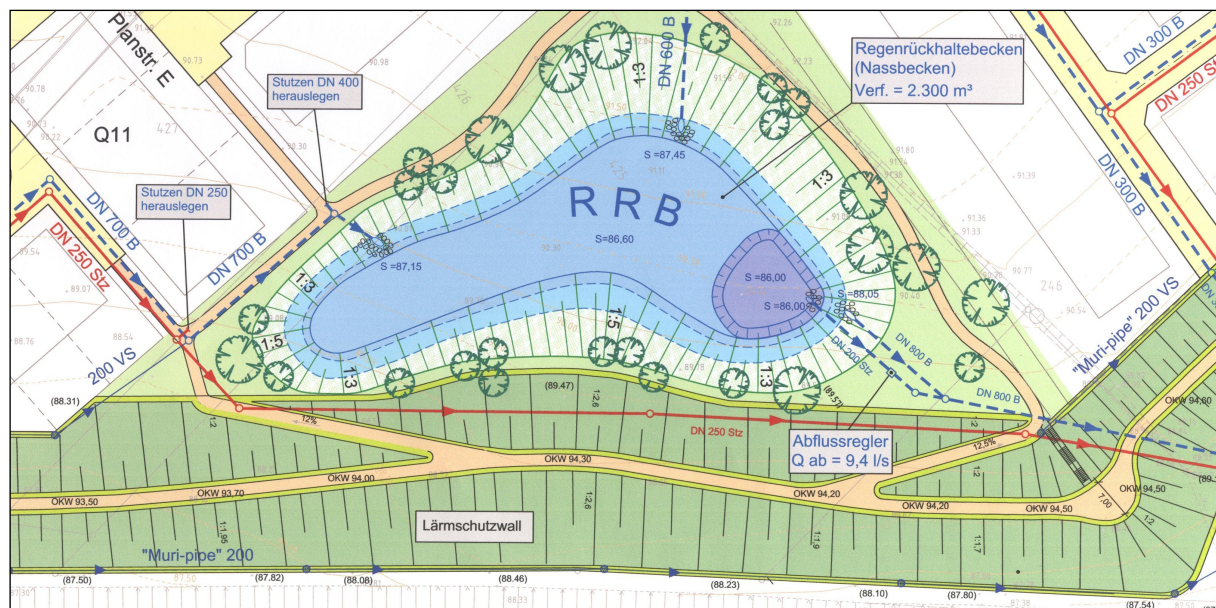
Regenrückhaltebecken
