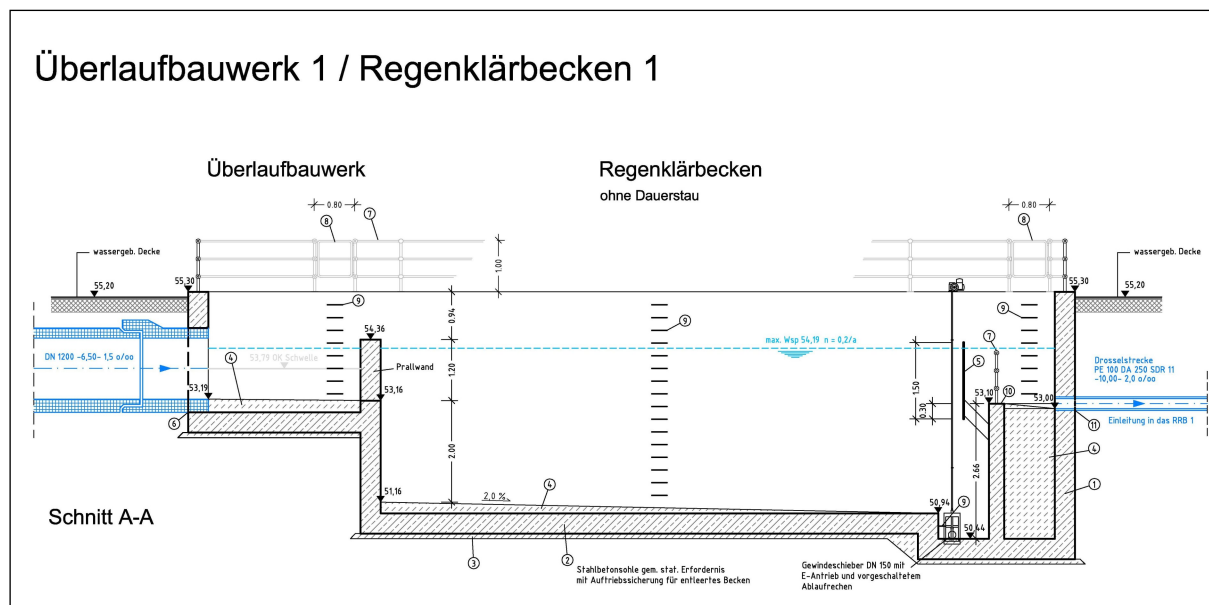
Überlaufbauwerk 1 / Regenklärbecken 1
