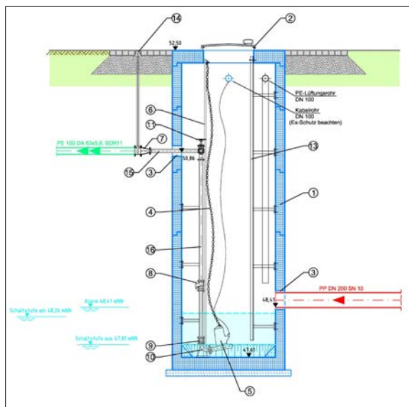
Schnitt Schmutzwasserpumpwerk
