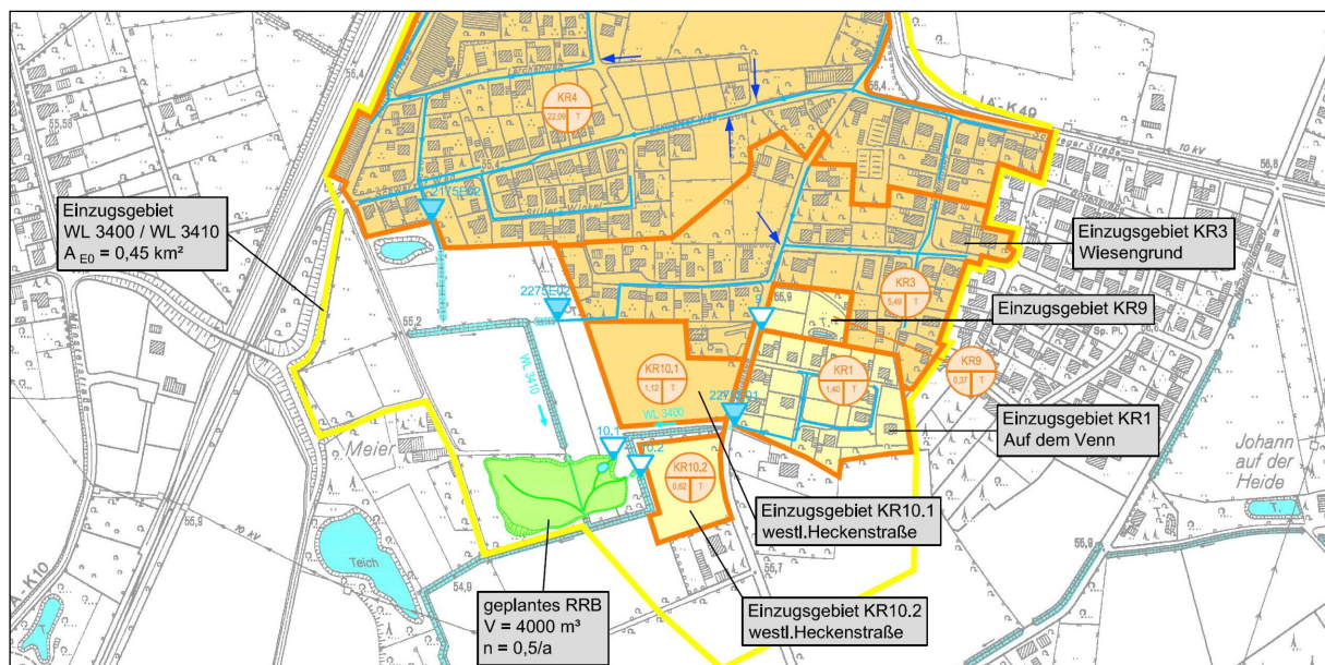
Ausschnitt Lageplan - Planung
